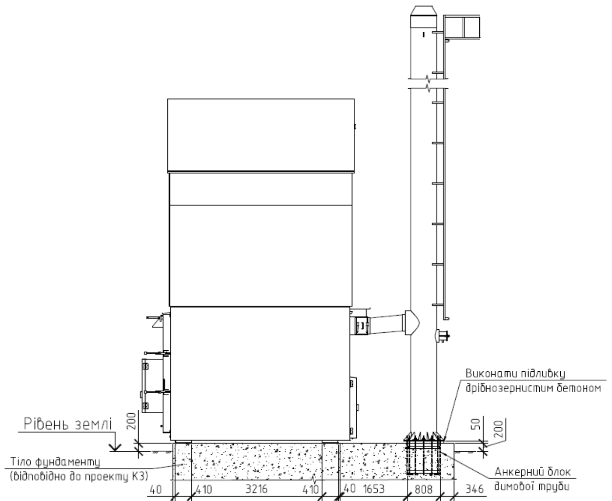
Мал. Схема фундаменту під теплогенератор.
